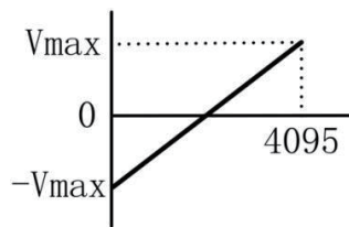
Fig. 2: Velocity linear mapping
